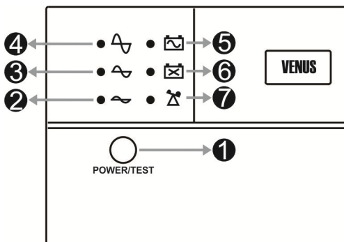
شکل ۲: نمای جلوی یوپی‌اس VENUS1300 (مدل ایستاده)
